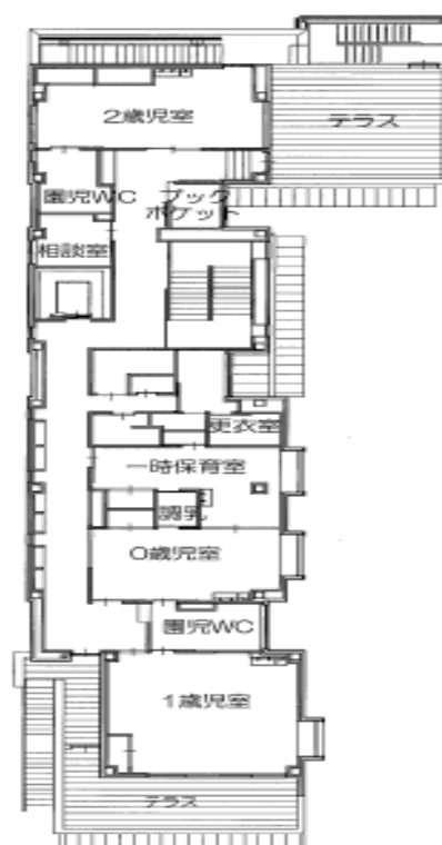
2階平面図
